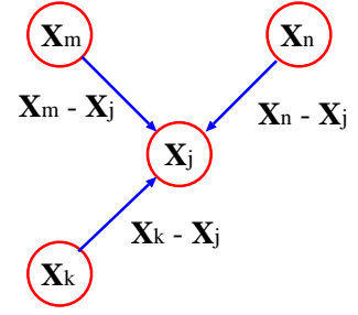
図2 ネットワークノード間の拡散。
