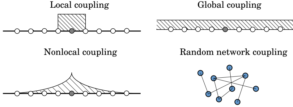
図5 典型的な結合ネットワーク.
