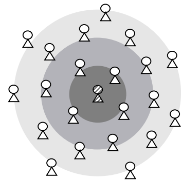
図1 自律要素の結合系。
