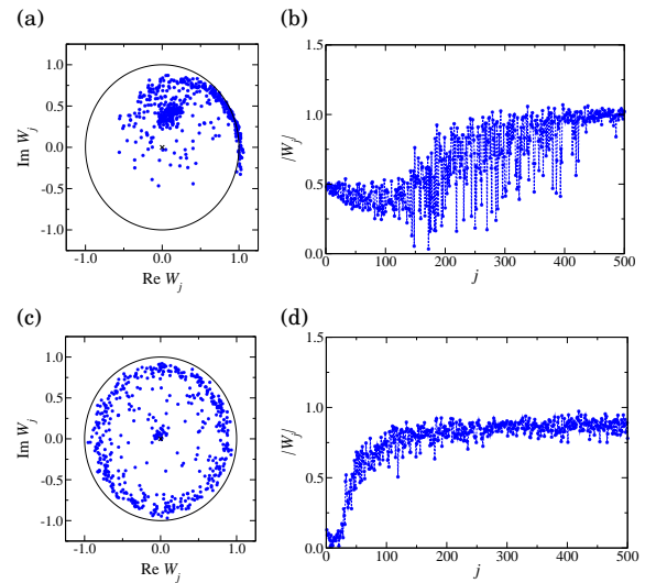
図 11 スケールフリーネットワーク結合 CGL 方程式. (a), (b): 結合強度 K = 0.02 で見られる部分振動停止状態, (c), (d): K = 0.04 で見られるカオス状態. (a),(c) は複素平面上的の振動子の状態 W_j のスナップショット, (b),(d) はノードに対して振幅の大きさ |W_j| のスナップショットをプロット。
