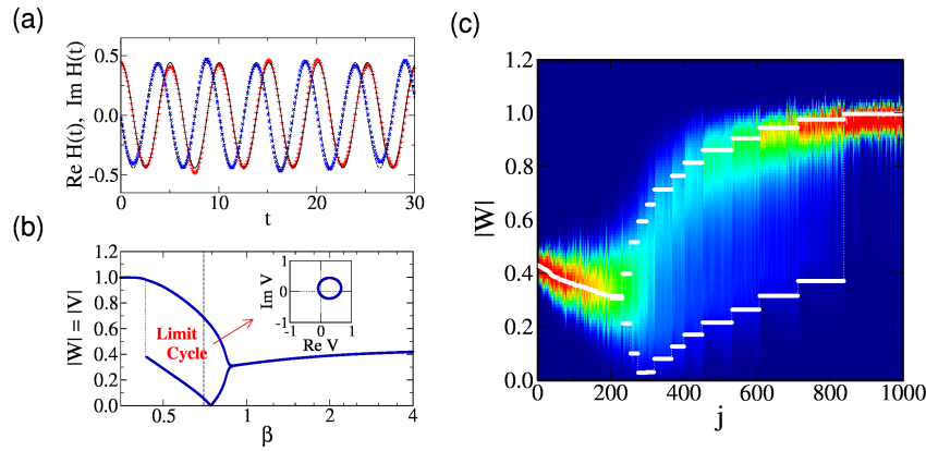
図6 CGLモデルの非一様パターンの平均場近似による理解 ( K = 0.04 ) . (a) ネットワーク上の大域平均場 H(t) の実部と虚部 (直接数値計算) . (b) 周期外力を受けた単一の振動子の分岐ダイアグラム . 複素振幅の絶対値 |W_j| の最大値と最小値を実効的な結合パラメータ \beta = Kk_j に対してプロット . (c) 直接数値計算によって得られた複素振幅の絶対値 |W_j| の分布と平均場近似の結果の比較 . 周期外力を受けた単一の振動子の分岐ダイアグラムをノード番号 j の関数として表示 .
