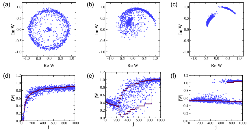
図5 スケールフリーネットワーク上の CGL モデルのダイナミクス (動的定常状態におけるスナップショット) . (a,d) 部分振幅停止状態 ( K = 0.02 ), (b,e) カオス状態 ( K = 0.04 ), (c,f) クラスター状態 ( K = 0.08 ) . (a),(b),(c) は全ての振動子の複素振幅 \{W_j\} の分布, (d),(e),(f) は振動子間の複素振幅の大きさ |W_j| をノード番号 j に対して表示 . (d),(e),(f) の実線は平均場近似によるもの .
