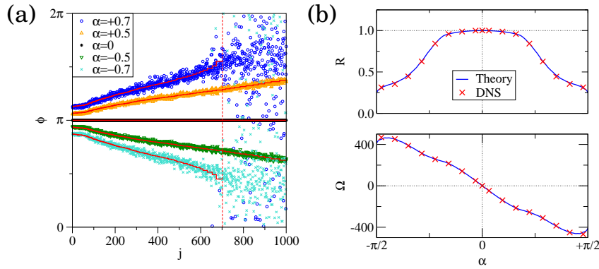
図4 ランダムスケールフリーネットワーク上の位相波．(a) 定常状態でのスナップショット．横軸はノード番号 (次数の大きい順にソート)． \omega = 1.0 , c = 5.0 , N = 1000 , \langle k \rangle = 20 で、いくつかの \alpha の値について表示．(b) 自己無撞着理論により得られた集団振動の振幅 R と振動数 \Omega を直接数値計算により得られた値と比較．横軸は \alpha で、 \alpha = 0 の時 \Omega = 0 となるように位相を定義している．
