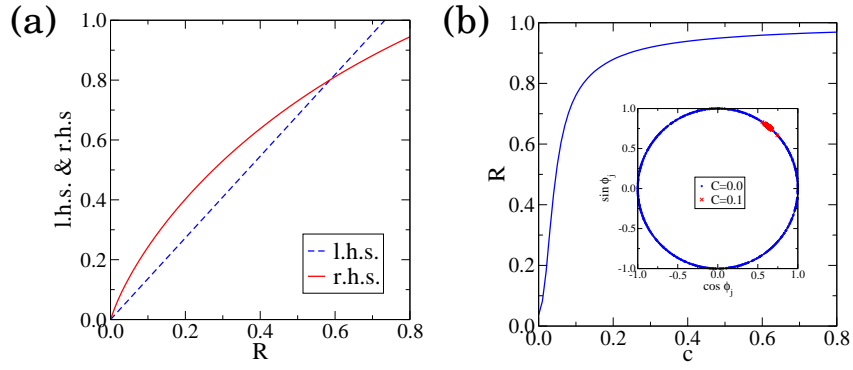
図3 (a) 自己無撞着な解析．自己無撞着条件の左辺と右辺が R > 0 で交われば，集団同期転移を示す． (b) スケールフリーネットワーク上の蔵本モデルの集団同期転移．結合強度 c と共に秩序パラメータ R が増大．挿入図は転移前 ( c = 0 ) と転移後 ( c = 0.1 ) での単位円上の振動子の分布．
