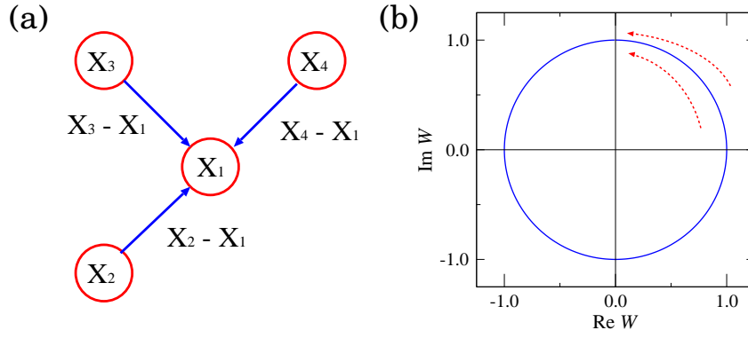
図 2 (a) ネットワーク上の拡散過程．化学物質等がノード間の濃度の差に比例して流れる．(b) 複素 Ginzburg-Landau モデルを構成する Stuart-Landau 振動子のリミットサイクル．複素平面上の原点が不安定化した固定点で単位円が安定なりミットサイクル軌道．
