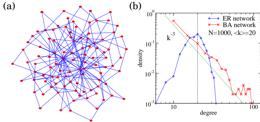
図 1 (a) Barabási-Albert のアルゴリズムで生成されたランダムスケールフリーネットワークの例．ネットワークサイズは N = 100 ，平均次数は \langle k \rangle = 4 ．極端に多くのエッジを持つハブが存在する．(b) Erdős-Rényi 単純ランダムネットワーク (ER) と Barabási-Albert スケールフリーネットワーク (BA) の次数分布の両対数プロット．いずれも N = 1000 ， \langle k \rangle = 20 ．ER ネットワークは平均次数の回りに次数分布が局在しているが，BA ネットワークはべき的で特徴的な次数がない．
