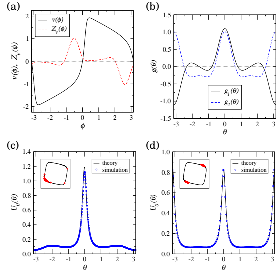
FitzHugh-南雲振動子の結果. (a) v(\phi) と Z_v(\phi) , (b) g_1(\theta) と g_2(\theta) , (c) 同期状態, (d) 2 クラスタ状態.
