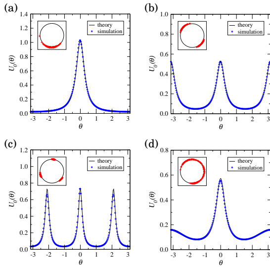
Stuart-Landau 振動子の結果. (a) 同期, (b) 2 クラスタ, (c) 3 クラスタ, (d) 混合状態.
